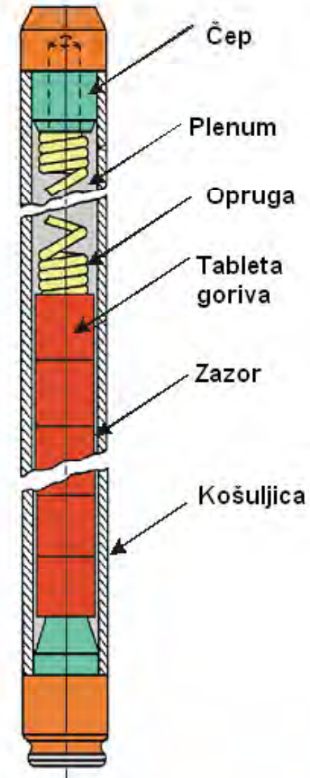
Gorivna šipka PWR reaktora
