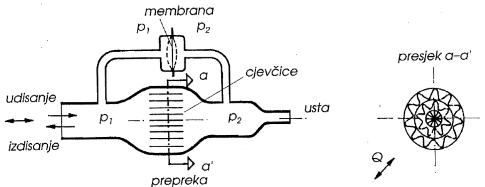
Slika 3. Spirometri otvorenog tipa s preprekom.
